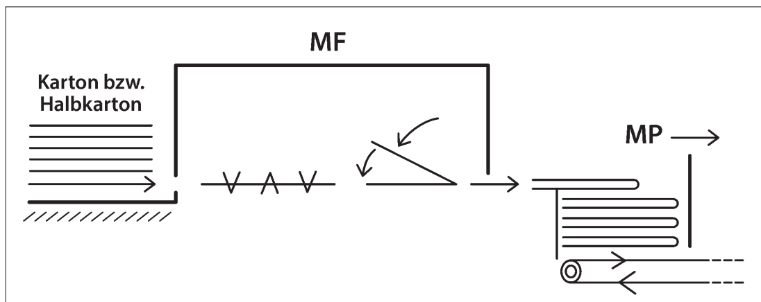
Funktionsschema des neuen FM+PM-Inline-Automats zur Tischkalenderfertigung der Swigraph AG.
