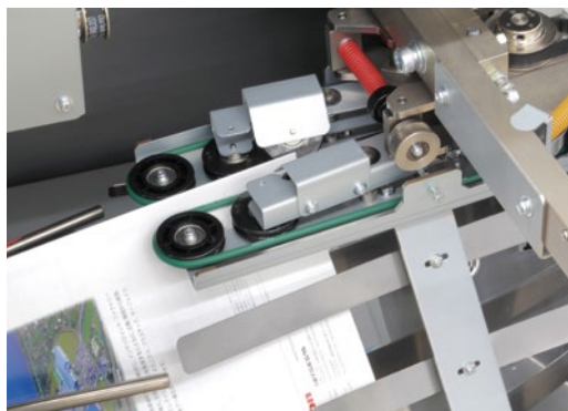
Beim Falzen erfolgen alle notwendigen Einstellungen für Format und Umfang selbstständig und präzise.
