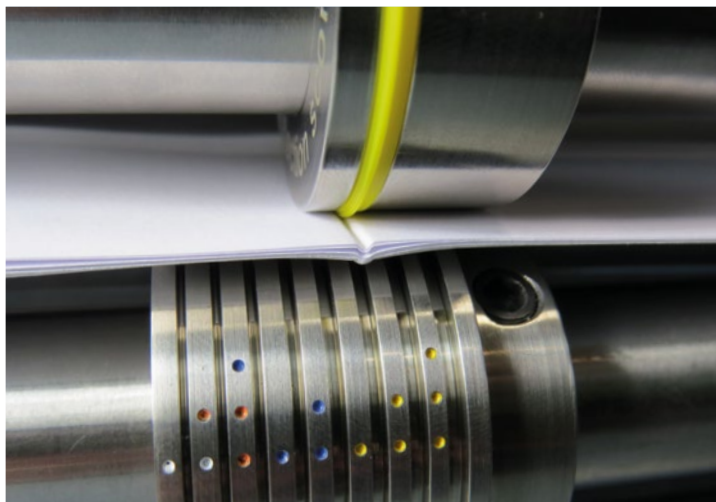
Mehrlagiges Papier zwischen Matrize und Patrize des Rillwerkzeugs Section Score. Uwe Reimold.
