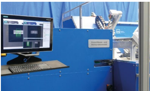
Das Ausschleuse- und Stichprobenmodul iChecker (l.) mit integriertem Kamerasystem prüft die Produkte während des laufenden Prozesses und kann fehlerhafte Exemplare automatisch ausschleusen. Der iPack (r.) im Showroom bei ETU.
